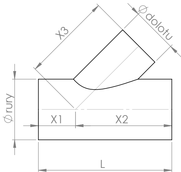
Trójnik pełny 45°
